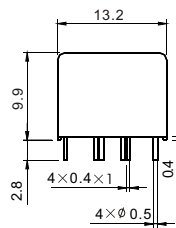
外形尺寸图
